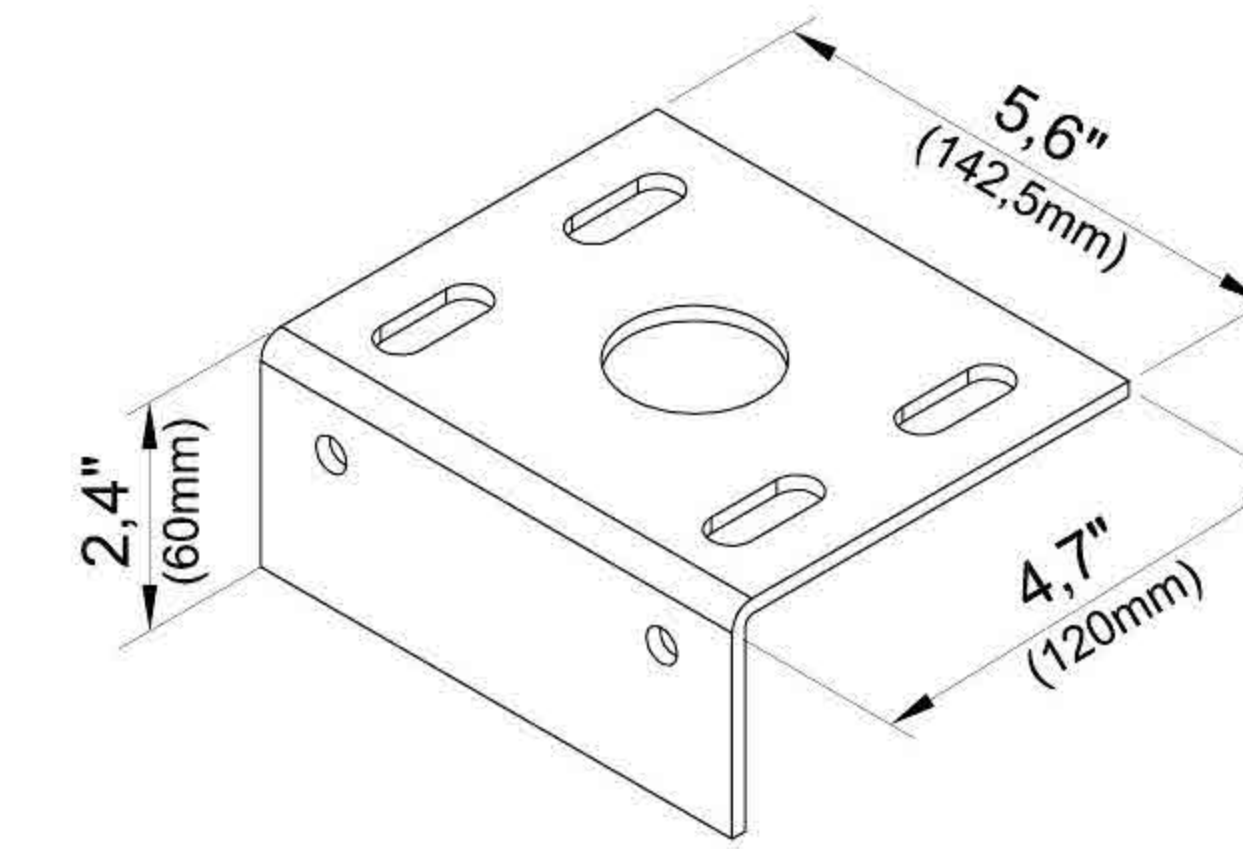
ZEMİN BAĞLANTI PLEYTİ İZOMETRİK GÖRÜNÜŞ
