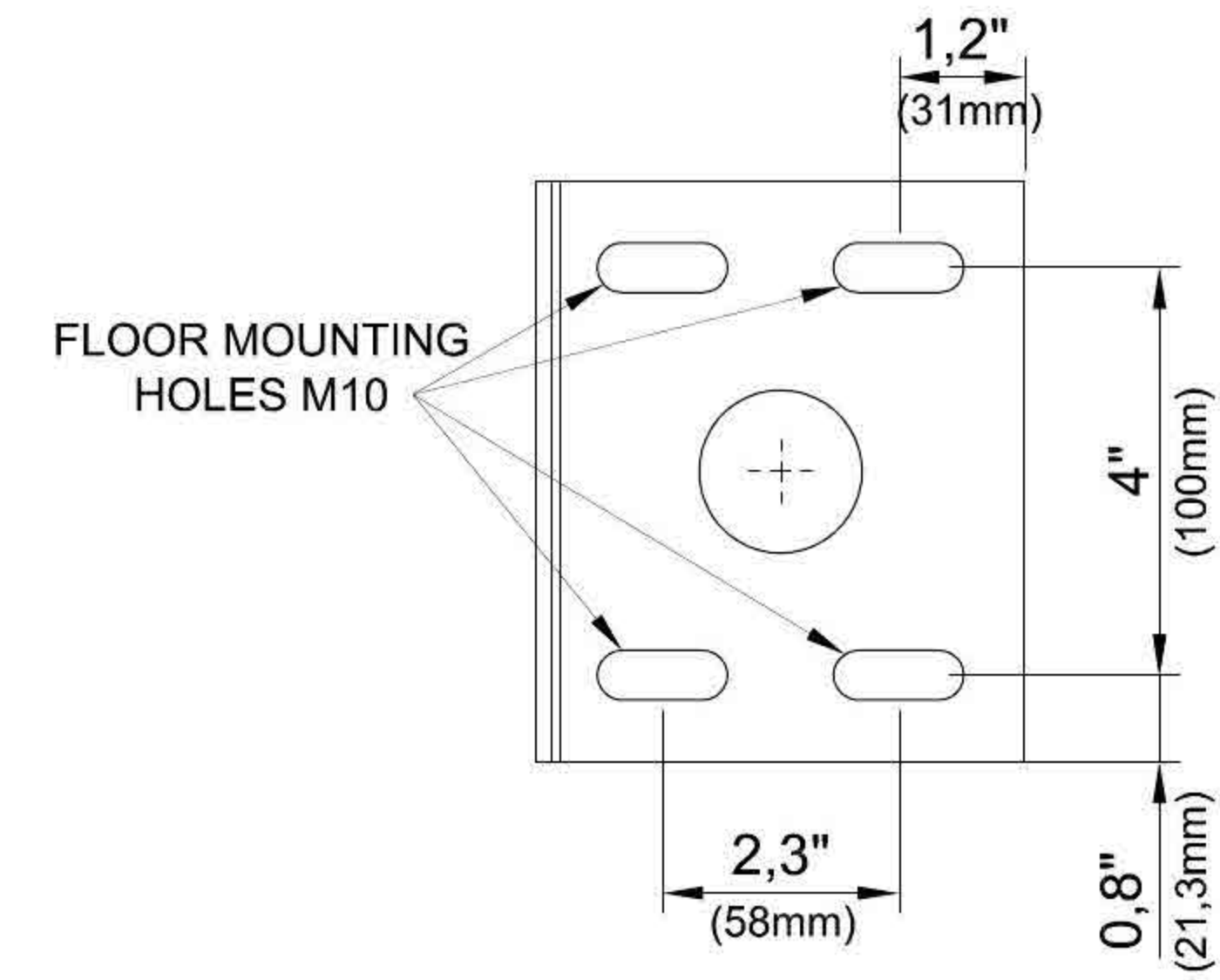
ZEMİN BAĞLANTI PLEYTİ ALT GÖRÜNÜŞ
