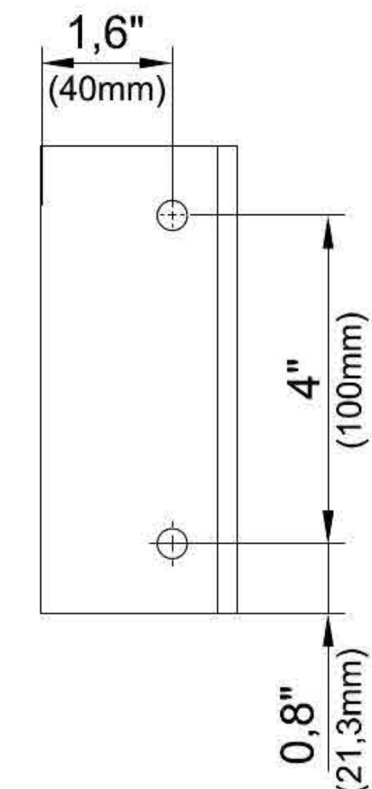
ZEMİN BAĞLANTI PLEYTİ ÖN GÖRÜNÜŞ
