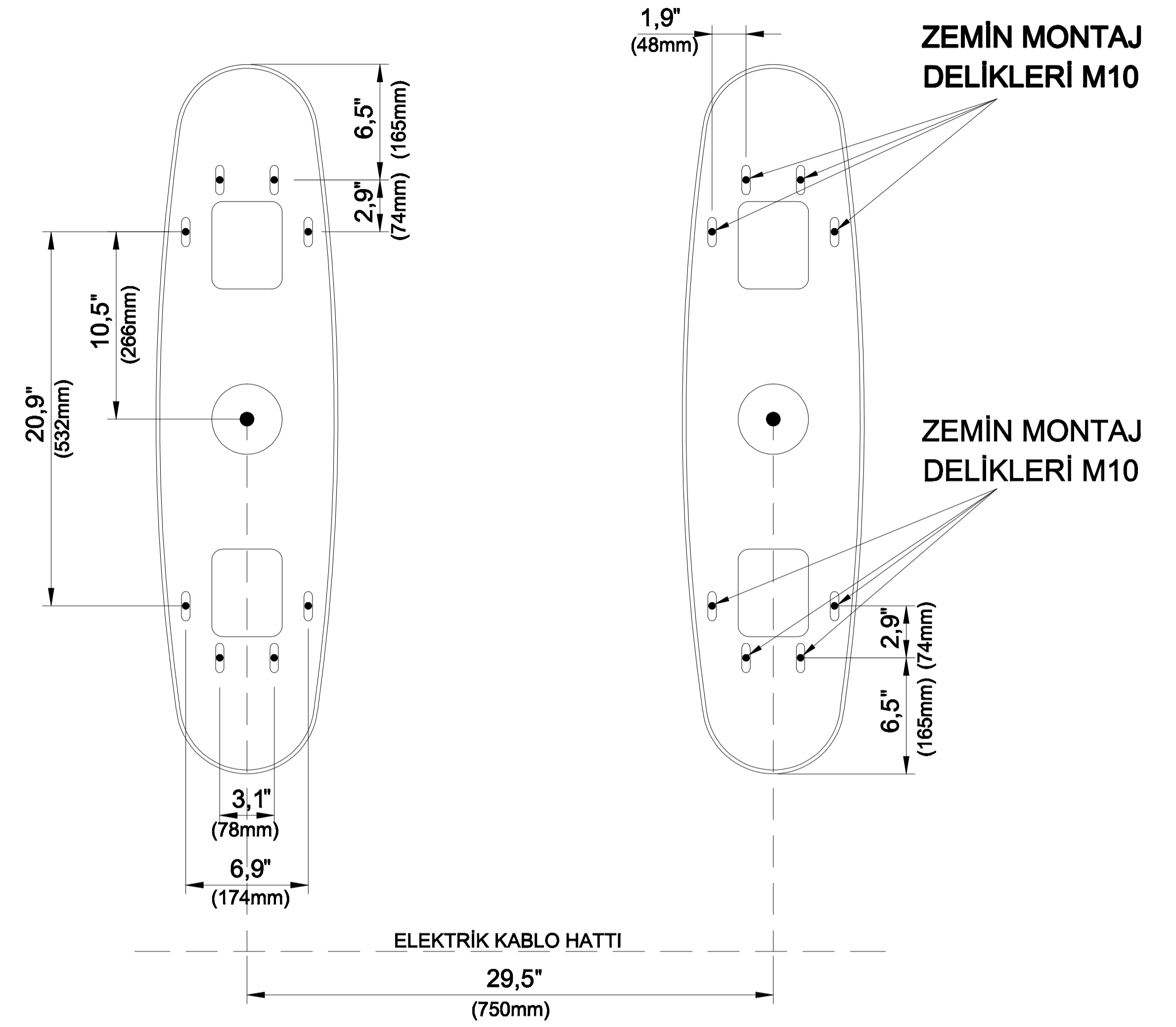
TURNİKE ALT GÖRÜNÜŞ
