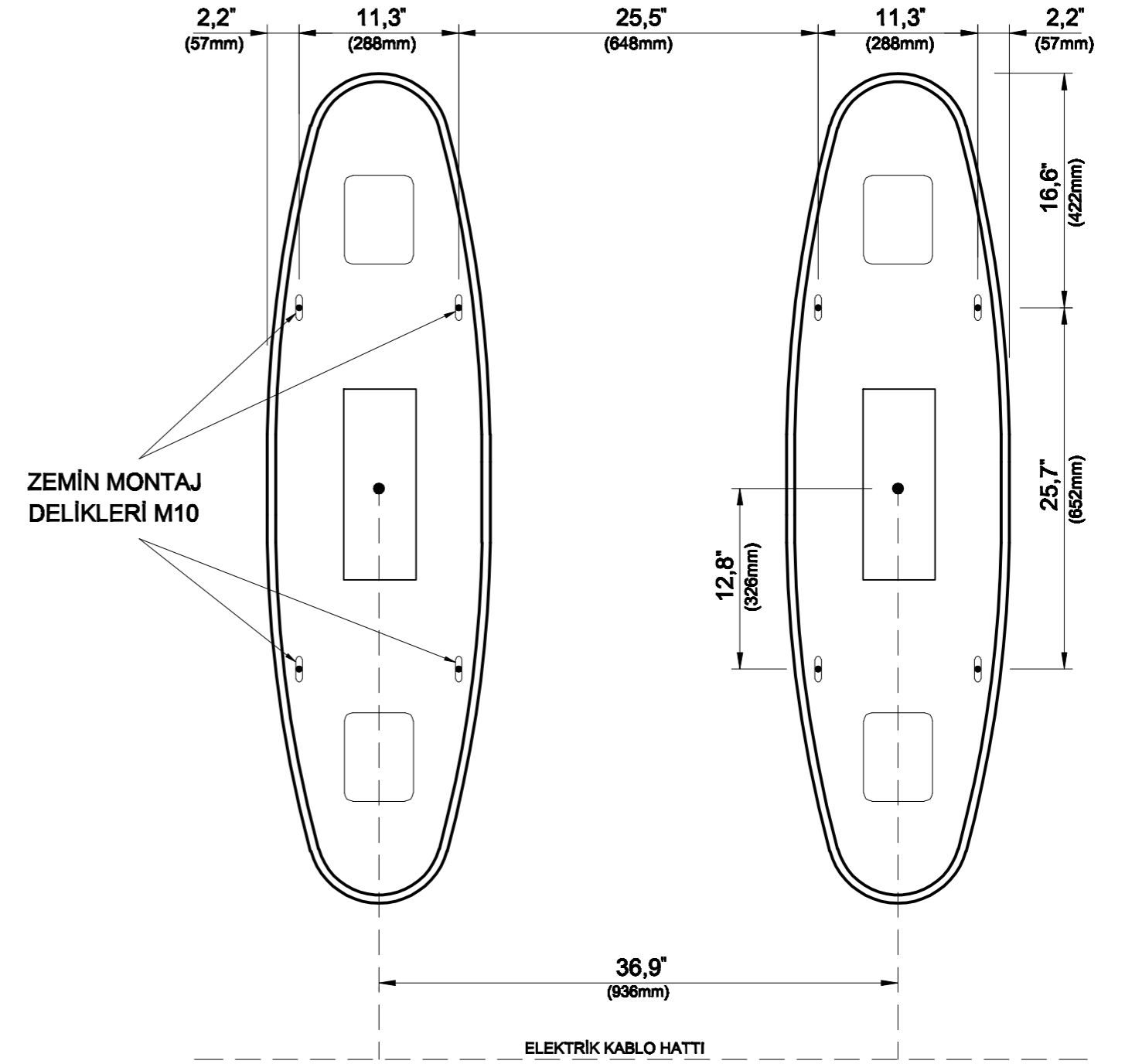
TURNİKE ALT GÖRÜNÜŞ
